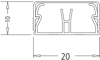
Dimensões Canaleta com divisória 20x10
