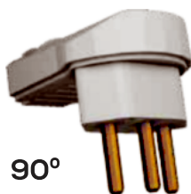
PLUGUE MACHO 2P+T 10A
