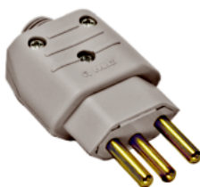
PLUGUE MACHO 2P+T 20A
