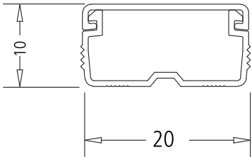
Dimensões Canaleta 20x10
