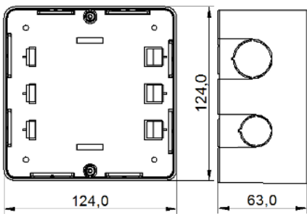
Dimensões Principais da Caixa (mm) 3213 / 3214
