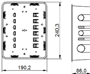
Dimensões Principais da Caixa (mm) 3215 / 3216
